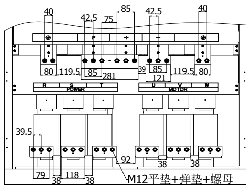
图 4-31: 500~630kW G3R 主回路端子 (机座号: A18)
