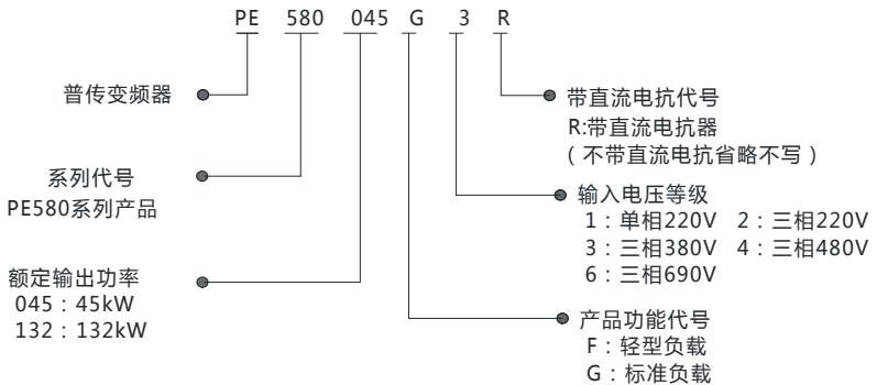
图 3-4 型号说明
