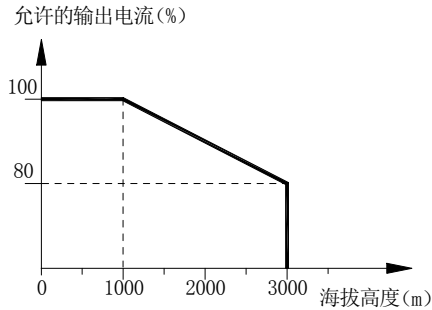
图 2-2: PE580 系列变频器超海拔降额曲线图
