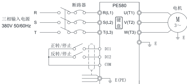
端子台控制电机正反转
