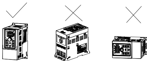
图 4-5：变频器安装示意图
