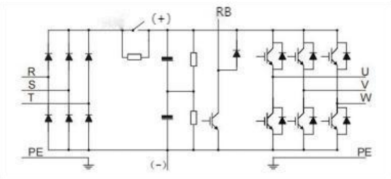
图 3-1 0.7~4kW 主回路简图
