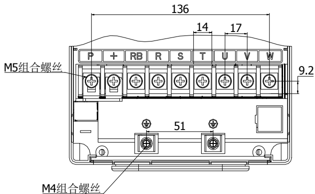
图 4-21： 15~22kW G3/F3 主回路端子图（机座号：A4）
