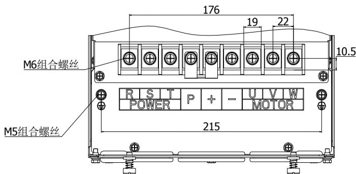
图 4-23: 37kW~45kW G3/F3 主回路端子图 (机座号: A6)
