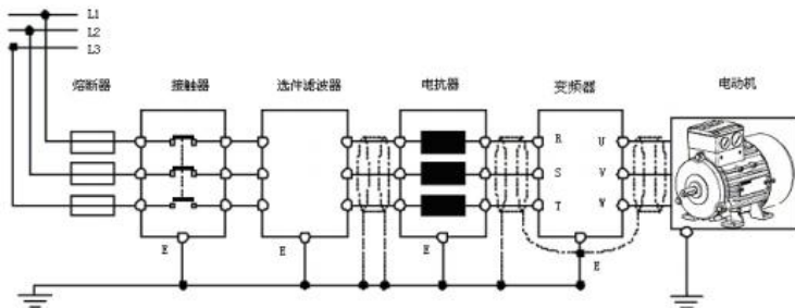
图 4-2: PE580 系列变频器系统接地图
