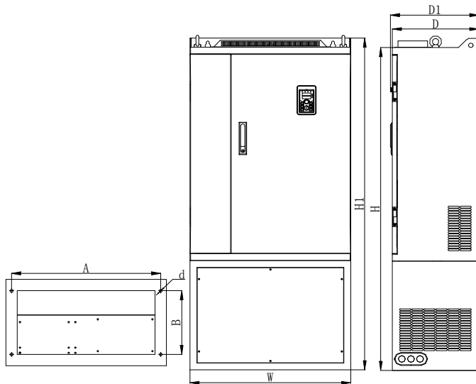
图 4-13： 132~220kW G3R（机座号：A13.1, A14~A15）
