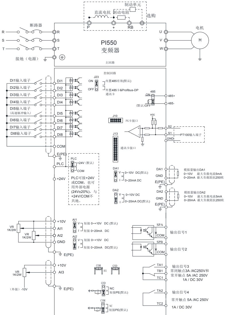
图 4-35：配线图
