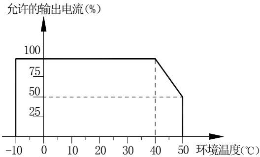
图 2-1: PE580 系列变频器超温降额曲线图
