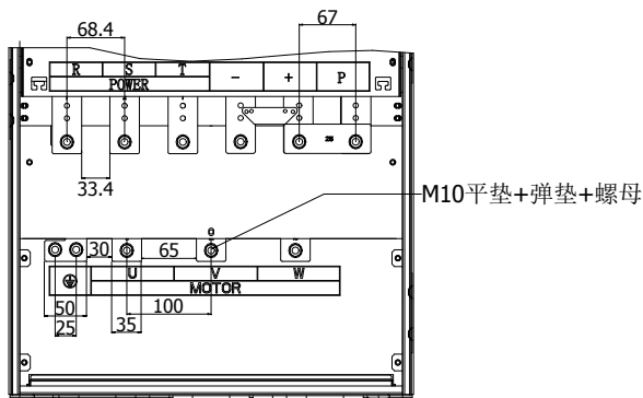
图 4-29: 187~220kW G3/F3 主回路端子 (机座号: A11)
