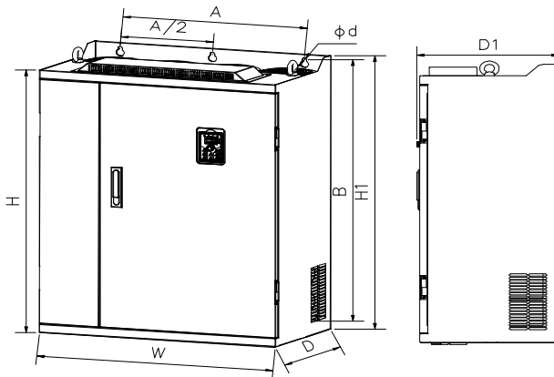
图 4-11: 30~220kW G3 外形尺寸 (机座号: A5~A11, A19)
