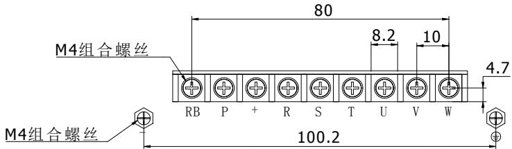
图 4-20： 5.5~11kW G3 主回路端子图（机座号：A3）
