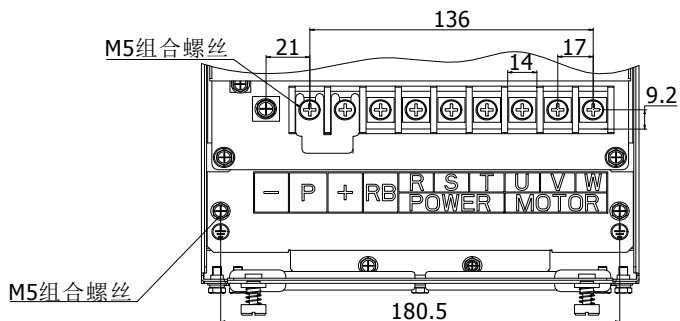
图 4-22: 30kW G3/F3 主回路端子图 (机座号: A5)
