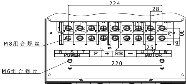
图 4-25: 75kW G3B 主回路端子 (机座号: A19)
