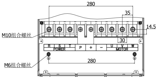
图 4-27: 93~132kW G3/F3 主回路端子图 (机座号: A9)
