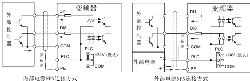
图 4-38：信号输入端子接线图—开路集电极 NPN 接线方式
