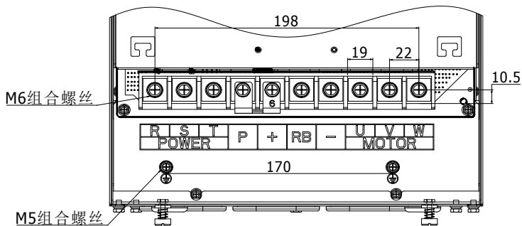
图 4-24: 37~55kW G3B 和 55kW G3/F3 主回路端子 (机座号: A7)
