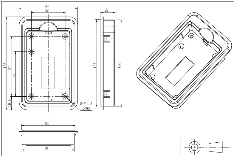
图 4-17: 键盘仓尺寸图 (尺寸单位: mm)
