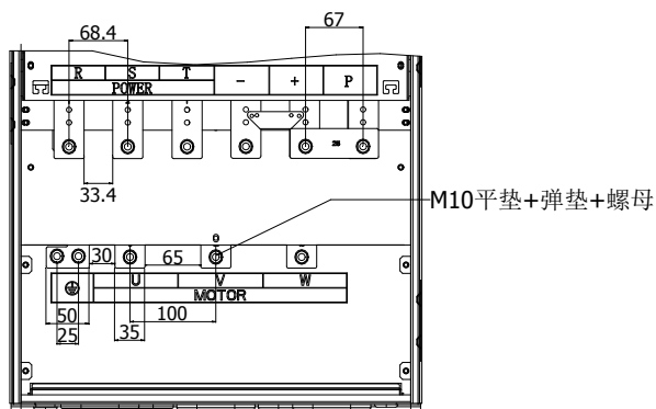
图 4-28: 160kW G3/F3 主回路端子 (机座号: A10)
