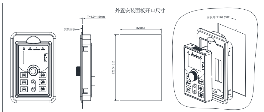
图 4-18： 键盘安装开口尺寸图(尺寸单位：mm)
