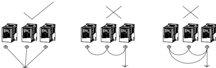
图 4-1: PE580 系列变频器多台并联接地图
