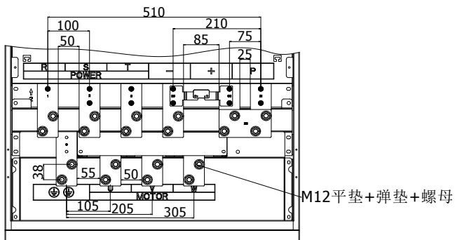
图 4-30: 250~450kW G3/F3 主回路端子 (机座号: A12~A13)
