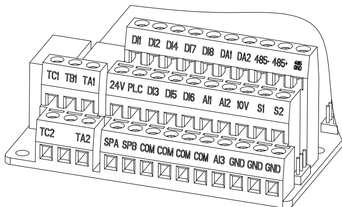
图 4-34： KZ12 控制板控制回路端子
