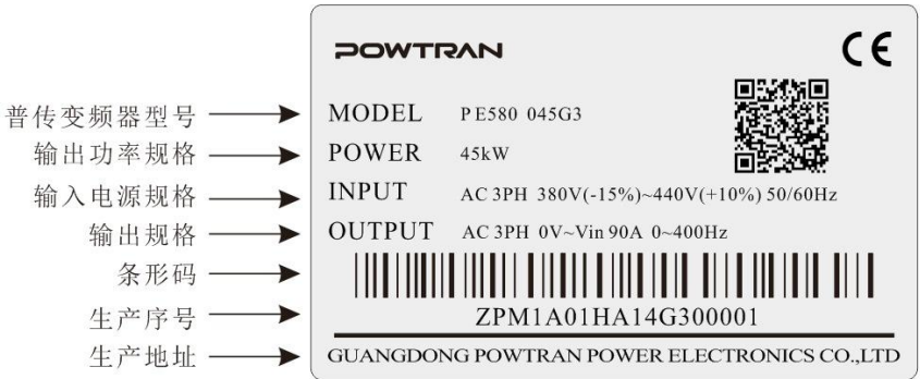
图 3-3 铭牌说明
