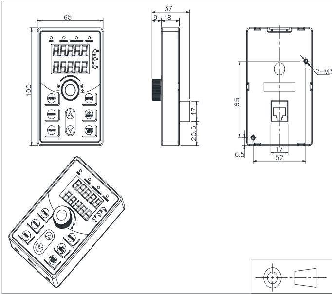
图 4-16: PE580 键盘尺寸图 (尺寸单位: mm)
