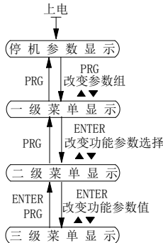
图 5-2：操作流程图
