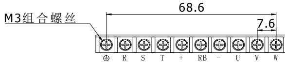
图 4-19： 0.75~4kW G3 主回路端子图（机座号：A1~A2）
