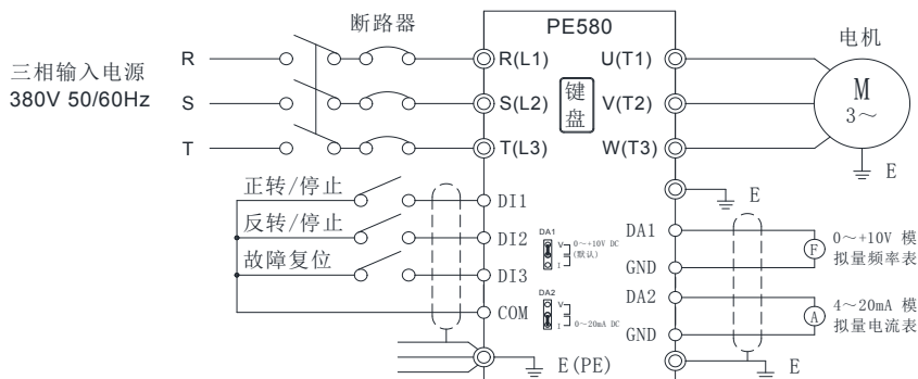
外接频率表与电流表
