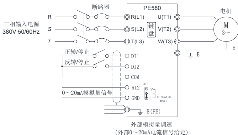
7-13-2 接法:
