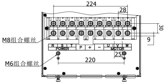
图 4-26: 75kW G3/F3 主回路端子图 (机座号: A8)
